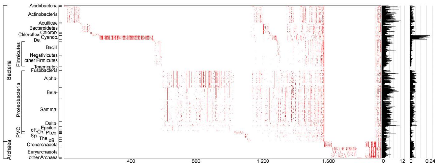
数据库统计分析： 功能基因的系统发生学模拟
